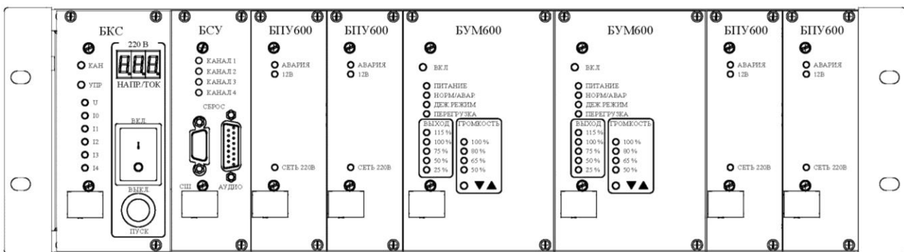
Вид спереди
