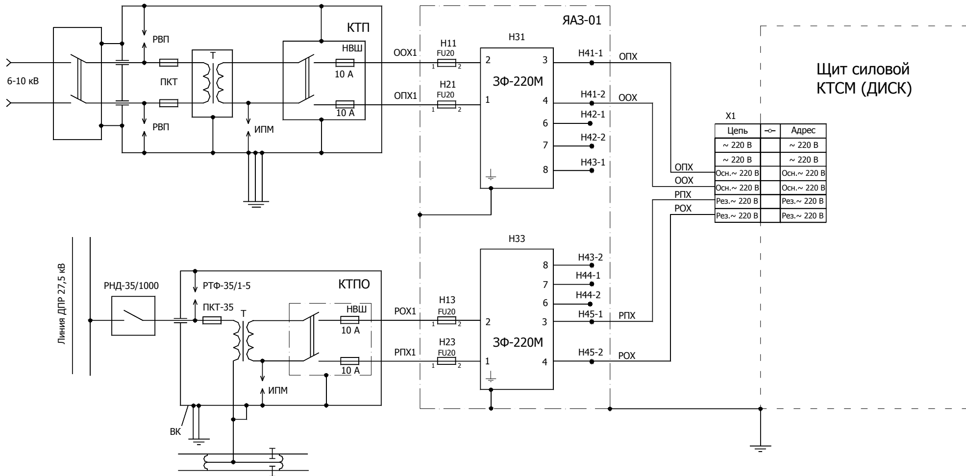
Рисунок 7. Схема включения защитного фильтра ЗФ-220М для защиты аппаратуры ДИСК и КТСМ при организации основного питания от КТП, а резервного от КТПО.
