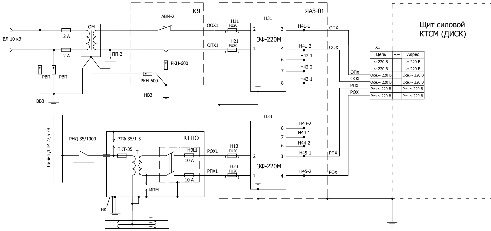
Рисунок 6. Схема включения защитного фильтра 3Ф-220М для защиты аппаратуры ДИСК и КТСМ при организации основного питания от трансформатора типа ОМ, а резервного от КТПО.
