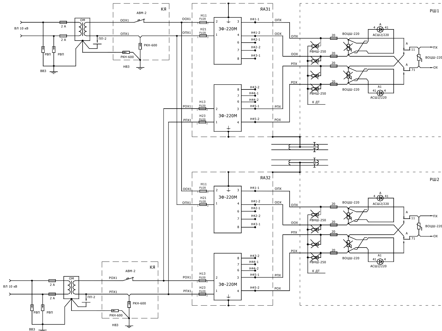
Рисунок 5. Схема включения защитного фильтра ЗФ-220 в составе кабельного ящика на спаренных сигнальных установках автоблокировки с размещением по разные стороны пути.
