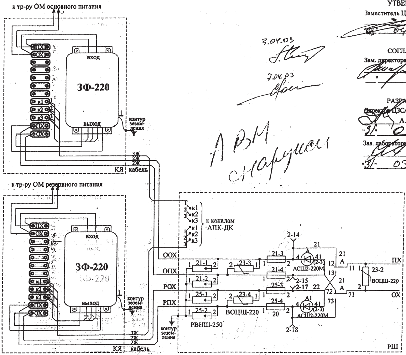
Схема включения кабельных ящиков с аппаратурой защиты 3Ф-220 по основному и резервному питанию на сигнальных установках автоблокировки.
